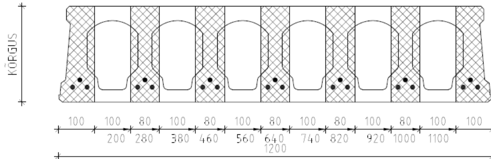
Joonis 1. Õõnespaneeli lubatud vertikaallõiked. Varjutatud tsoonis lõikamine ei ole lubatud.
